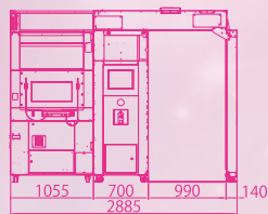
側面図
